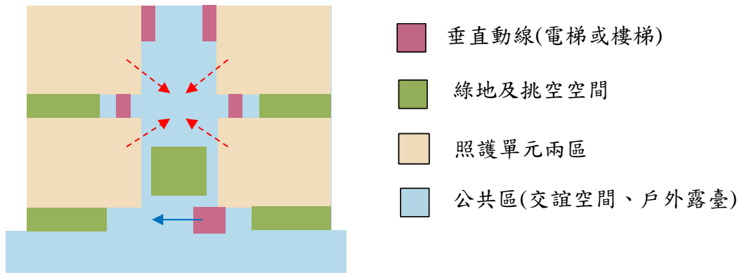
圖6 三層平面
